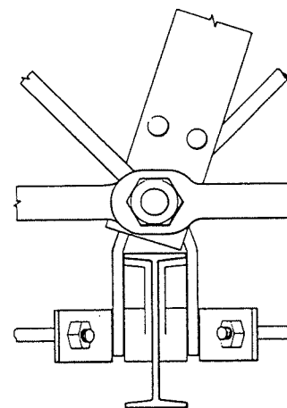
Elevation L4
