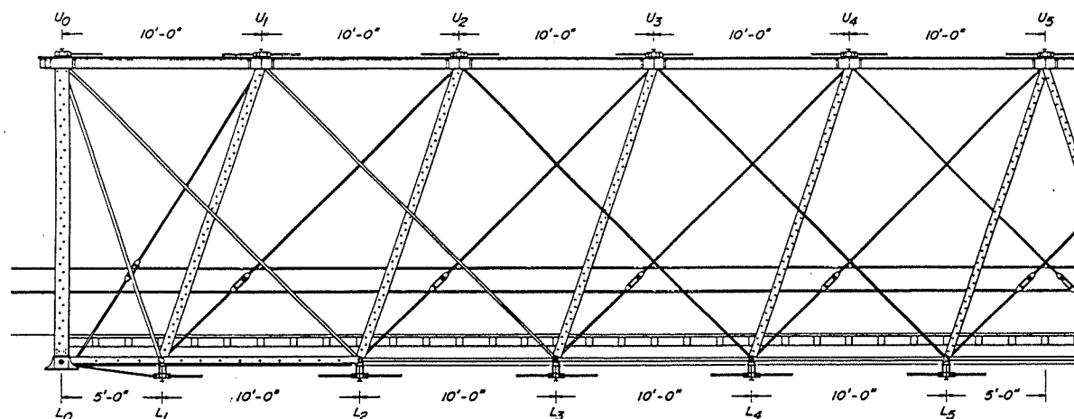
Elevation
