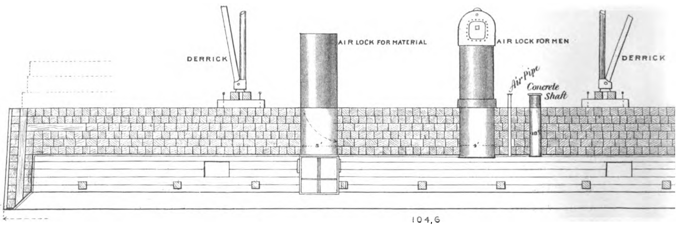
LONGITUDINAL SECTION
