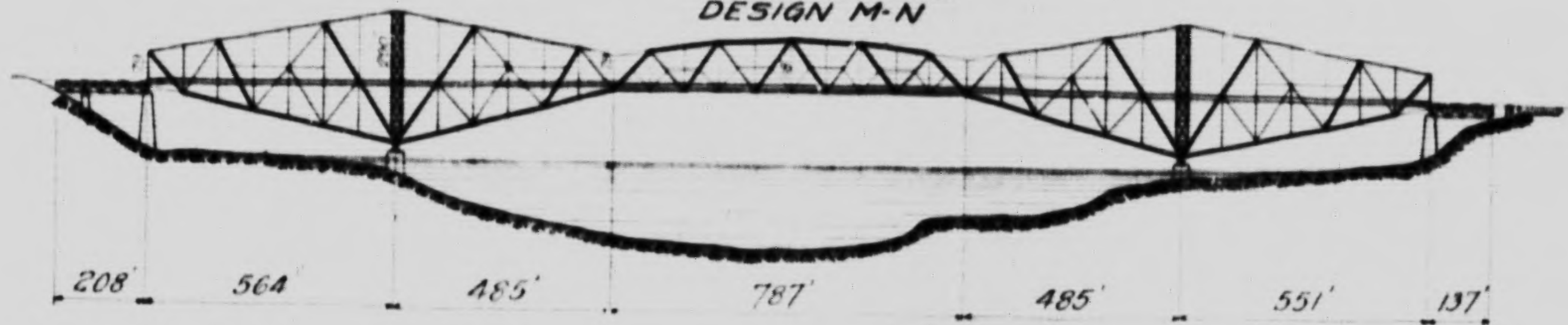
FIG 6 MASCHINENFABRIK AUGSBURG-NÜRNBERG A.G. QUEBEC BRIDGE.
