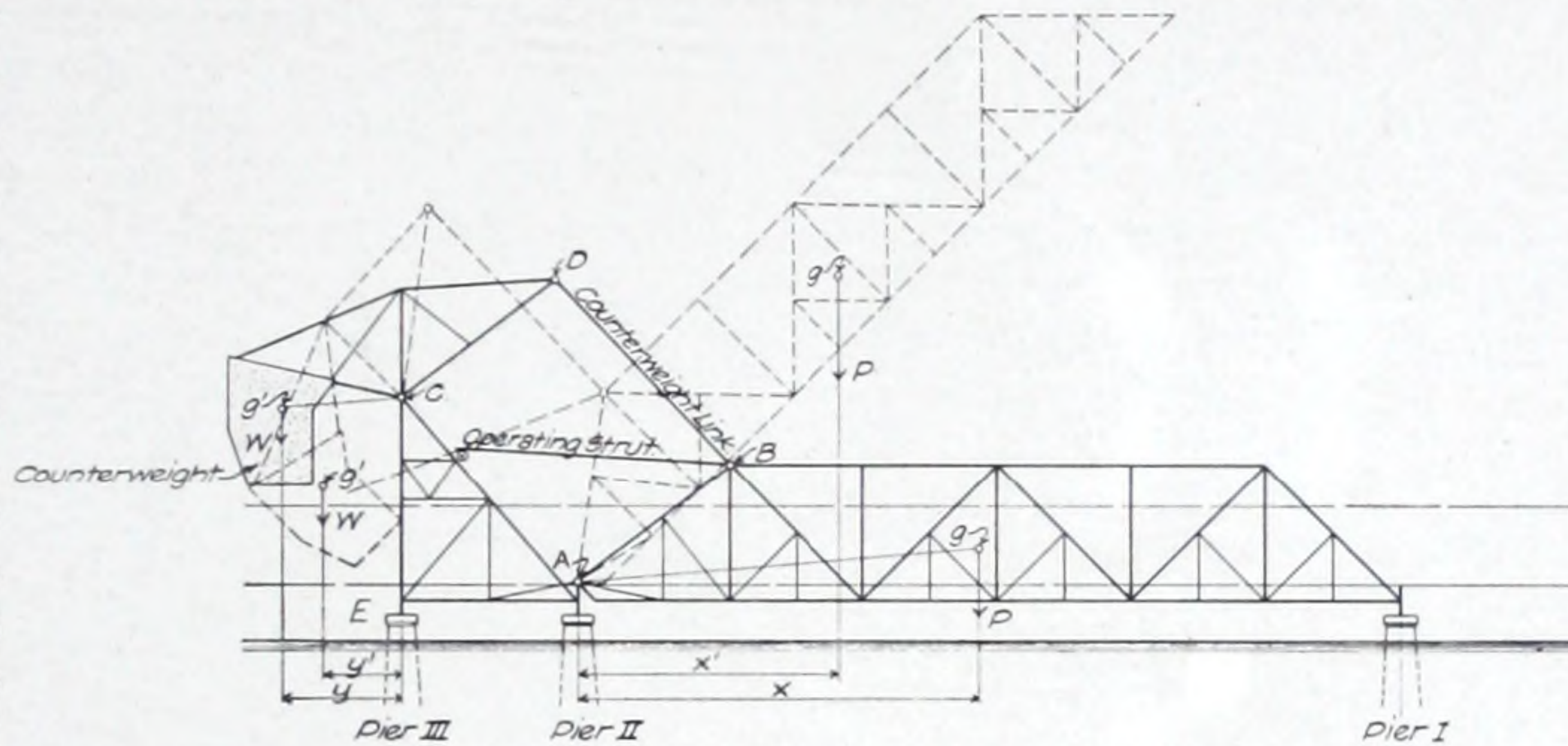
FIG. 18. DIAGRAM HEEL TRUNNION TYPE.
