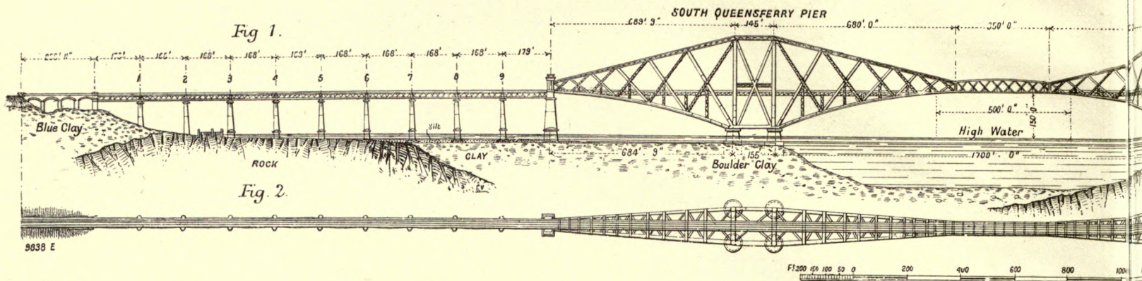
Fig. 16. Trestle
